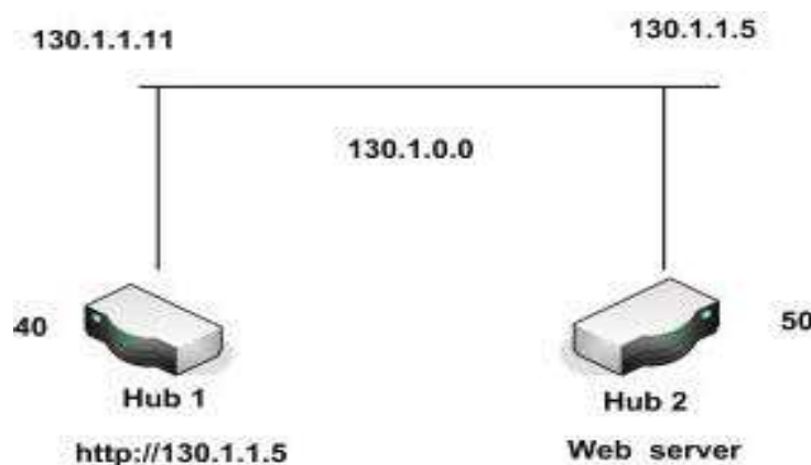
شکل ۲۷: مثالی از ارسال یک بسته TCP/IP
